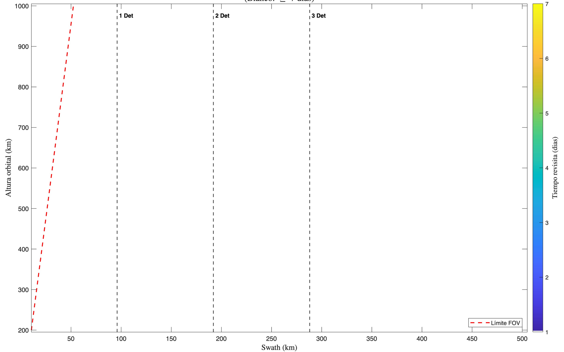
Tiempo Revisita - 2 Satellite(s); 1 Telescopio(s): Cassegrain; Detector 1 (Blanco: \geq 7 días)
